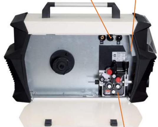
4-kladkový posuv 4-rolls wire feedern
